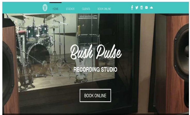
Kuva 7. Musiikkistudion www-sivut
