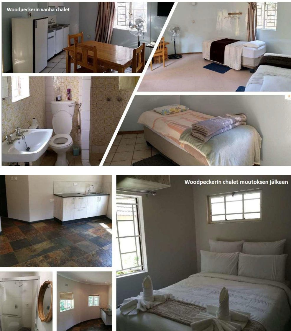
Kuva 5. Woodpeckerin chalet
